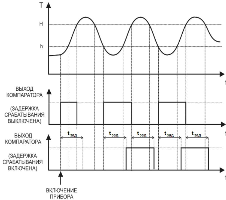
Рисунок 6 – Временная диаграмма работы компаратора с заданной задержкой срабатывания
