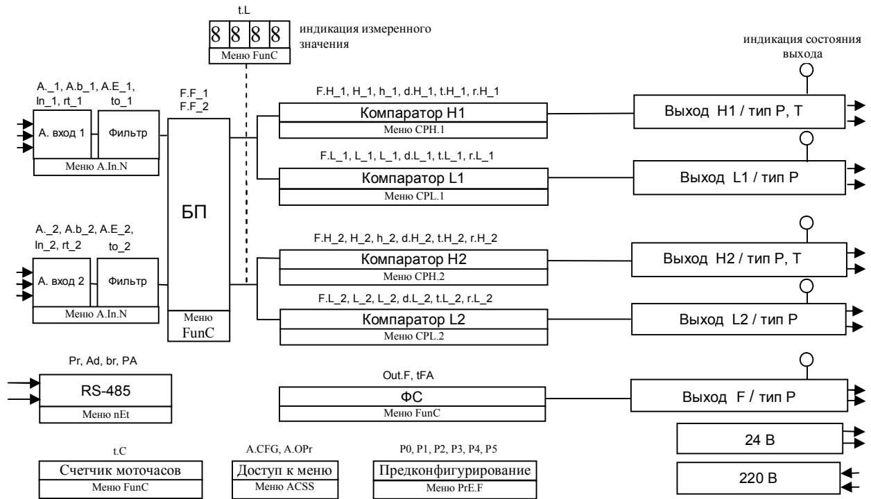
Рисунок 2 – Функциональная структура приборов M-1725-2P/2P, 2T/2P
