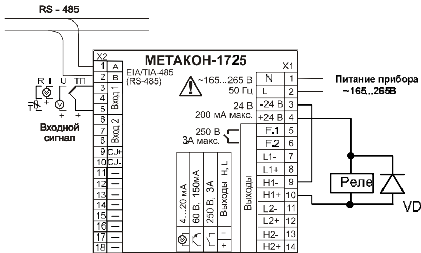
Рисунок 10 – Электрическая схема подключения к прибору МЕТАКОН–1725–2Т/2Р–1 при использовании встроенного источника 24 В для питания внешнего промежуточного реле, подключенного к открытому коллектору оптотранзистора
